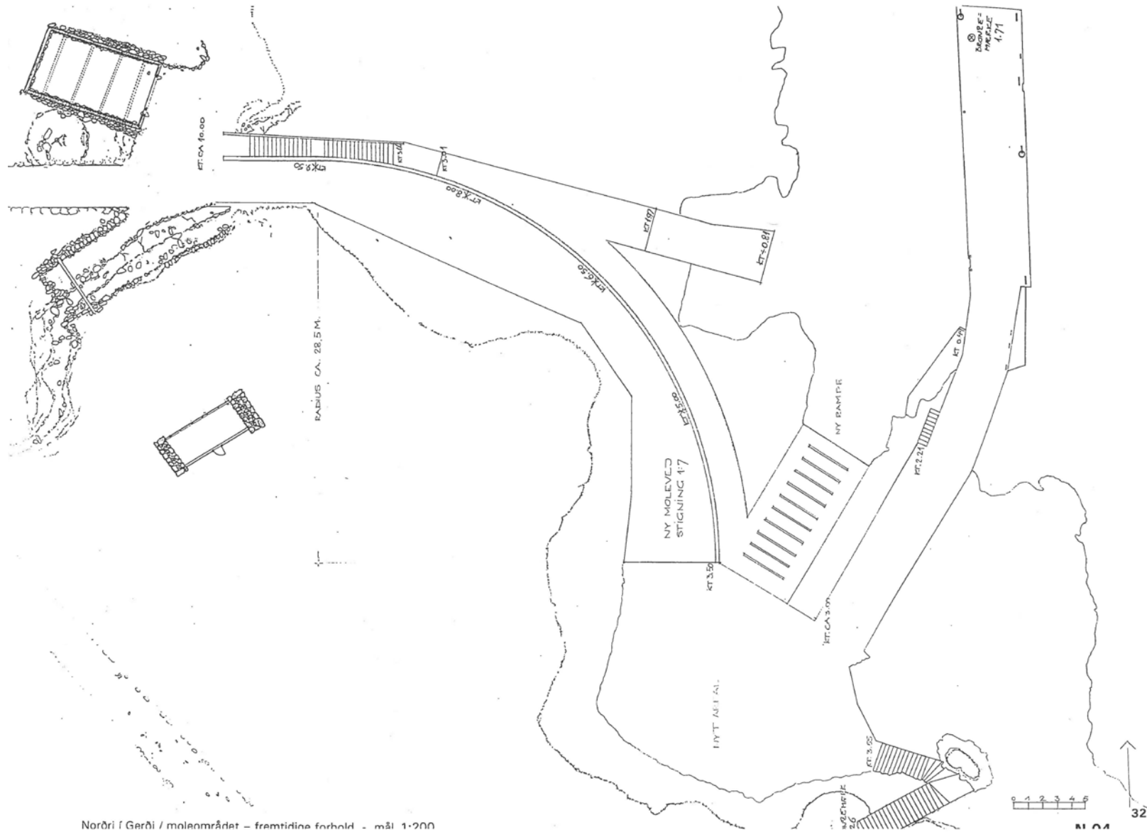
Norðri / Gerði / molemráðet - fremtidine forbold - mál 1:200
