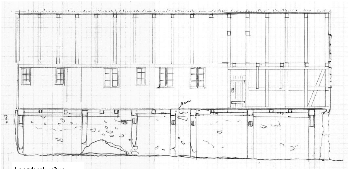
Longdarskurður
