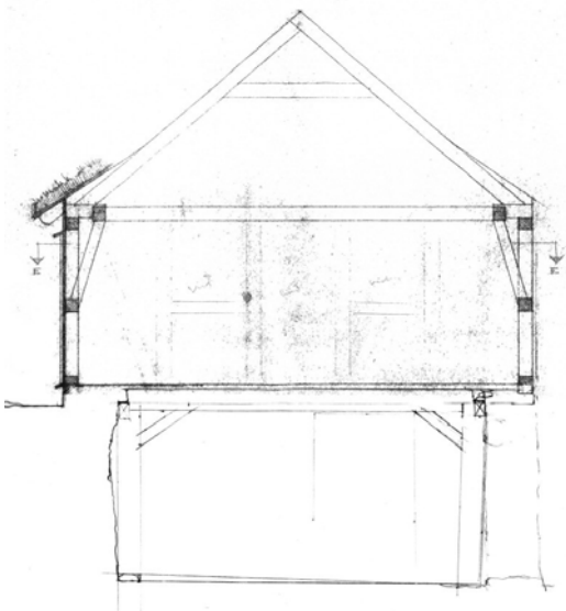
Tvørskurður
