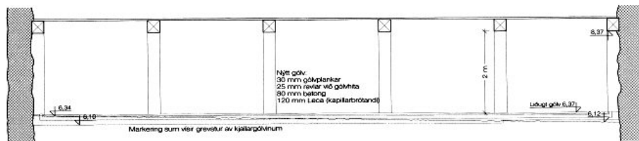
Prinsipp-longdarskurður
