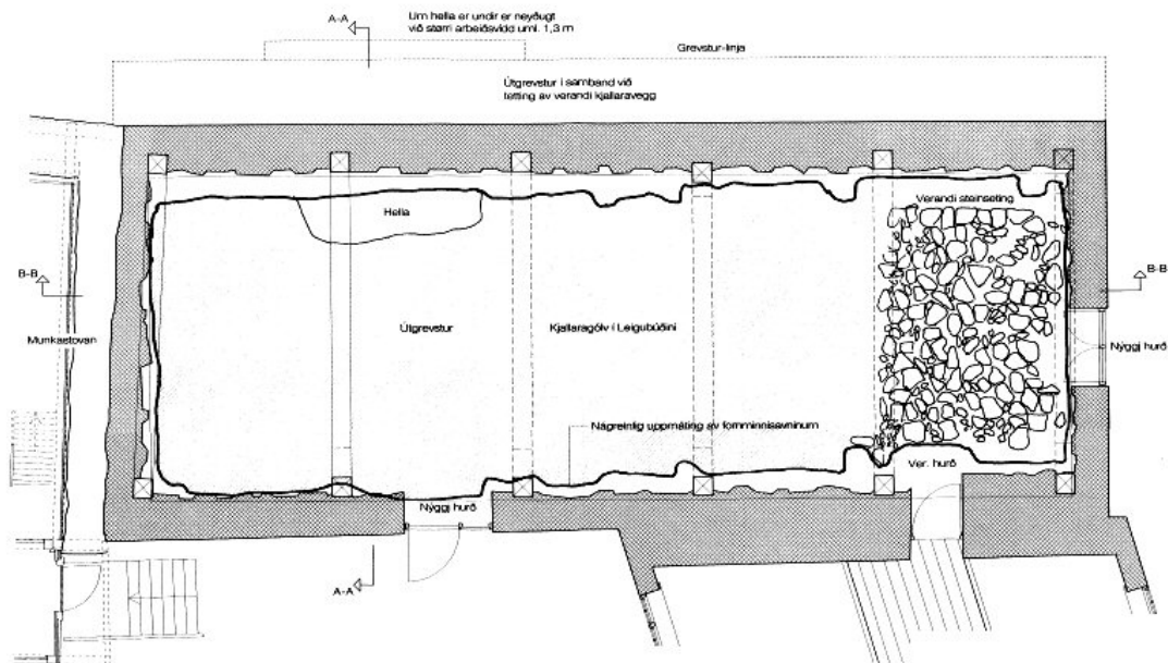
Kjallarahædd
