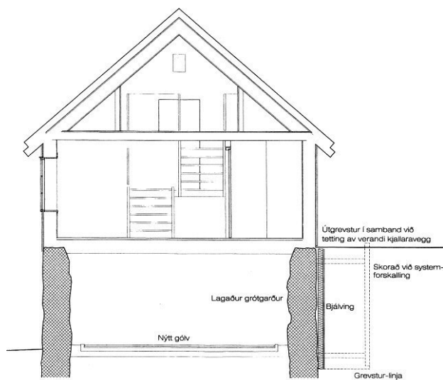
Tvørskurður A-A
